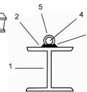
d) Ancre structurelle avec point d'ancrage
